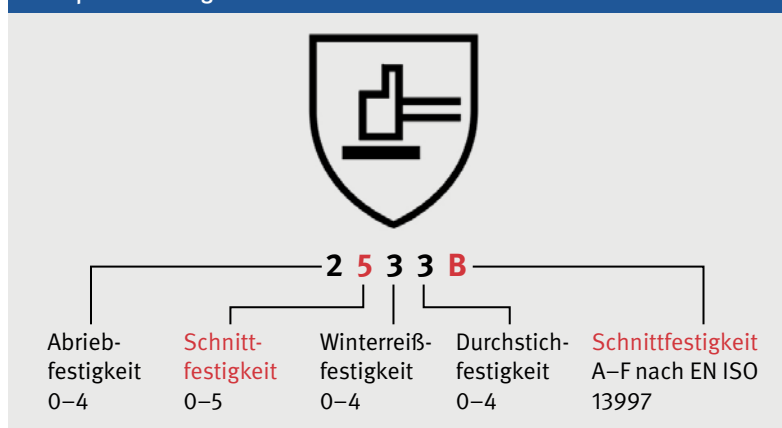
Beispiel: Leistungsstufen Schnittschutz nach DIN EN 388
